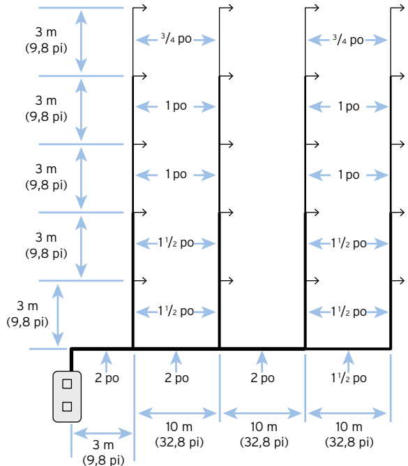
Schéma 4 - Diamètres et longueurs des sections du réseau de distribution d'eau chaude
