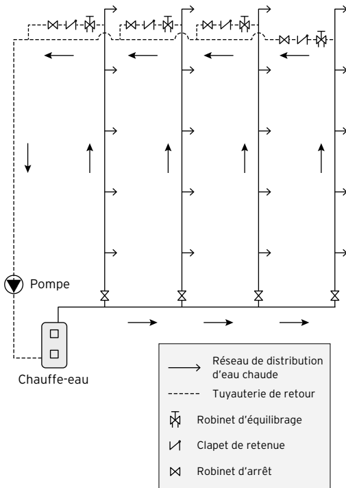
Schéma 3 - Exemple d'agencement pour un immeuble à logements
