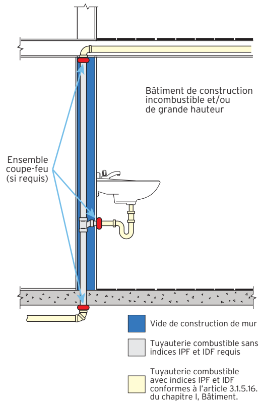
Schéma 4 - Tuyauterie combustible logée dans un vide de construction d'un mur
